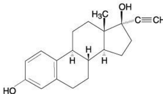
Ethinyl estradiol
